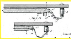
1914 Brevet Wiegand, tube avec résistance droite isolée magnésie.
