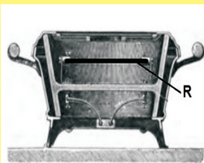
1899 Résistance chauffante métal-céramique Parvillée (document Ultimheat Museum)
